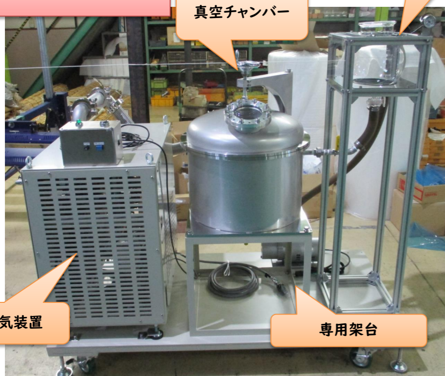
真空チャンバーセット商品 製作事例①
