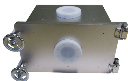
横扉ステンレス真空チャンバー（小型） W:420×D:300×H:260
