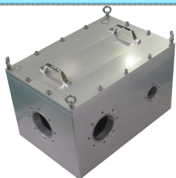
上蓋アルミ真空チャンバー W:600×D:400×H:365
