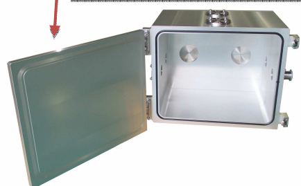
横扉アルミ真空チャンバー W:620×D:450×H:520
