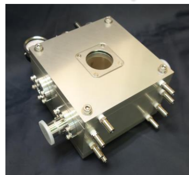
アルミ真空チャンバー W:190×D:190×H:120
