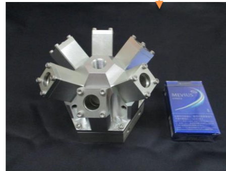
小型アルミ真空チャンバー W:95×D:110×H:110
